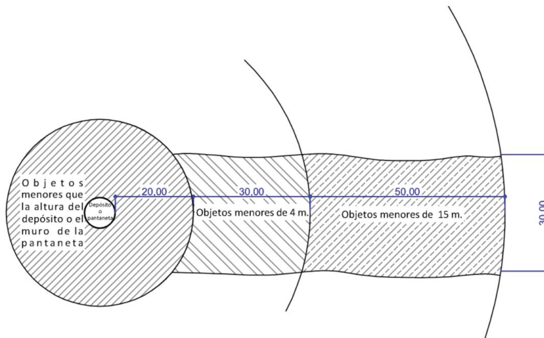
Figura 4. Planta de características de zona con depósito de agua o pantaneta.
